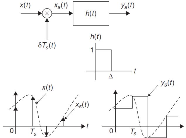
Figura 15. Muestro utilizando un sistema de muestreo y retención
